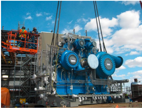
Montage eines CO 2 -Verdichters.
